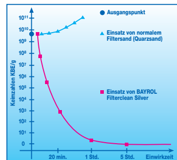
Keimtötung bzw. Keimwachstum bei abgeschalteter Umwälzpumpe (Modellversuch).
